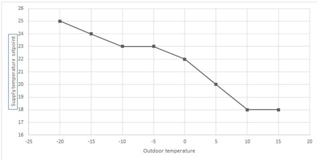
Bild 4-2 Temperatur-Kompensationskurve
