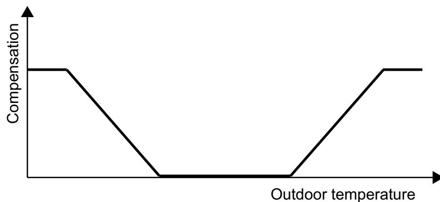
Bild 4-12 Beispiel für die Ventilatorkompensationskurve
