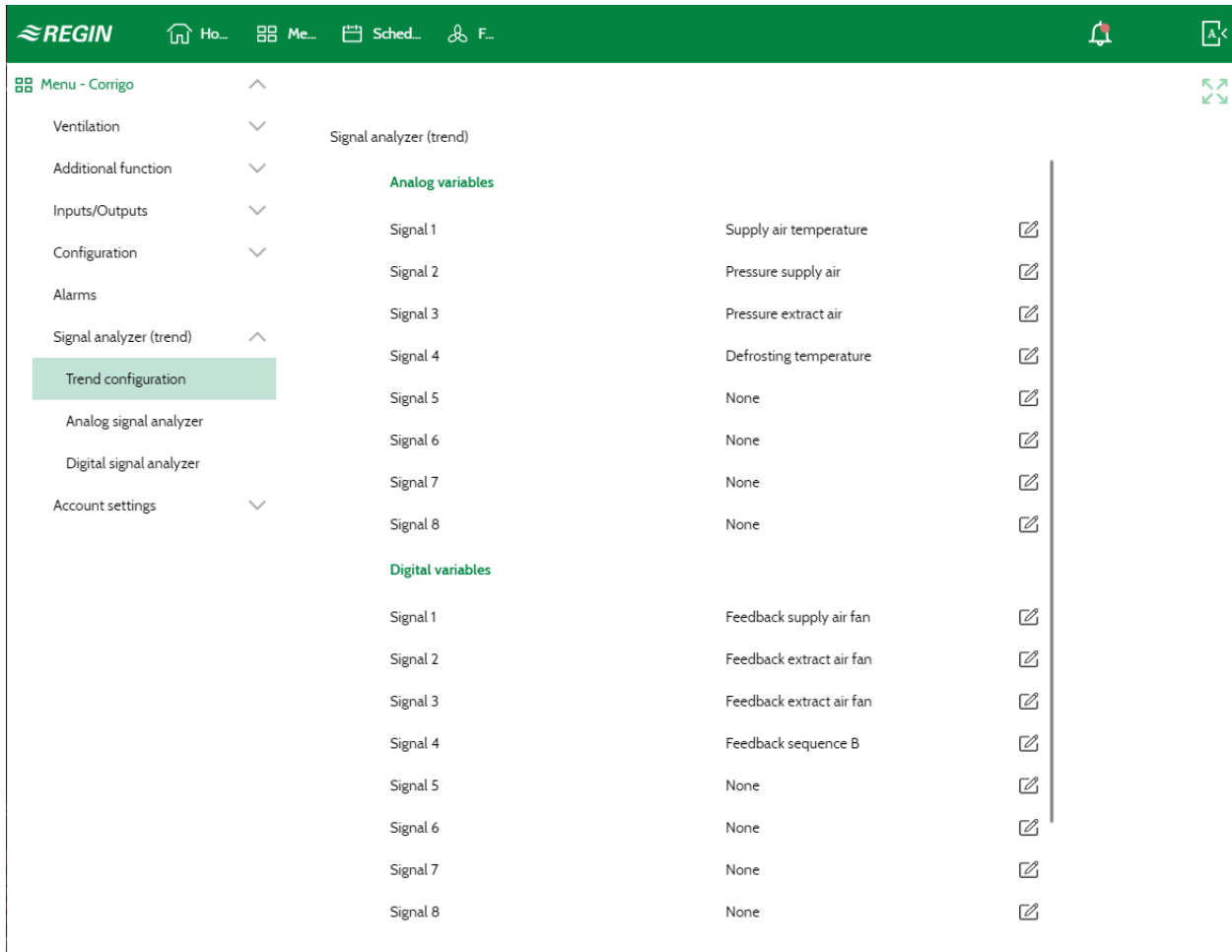
Bild 3-12 Konfiguration des Signalanalysators
