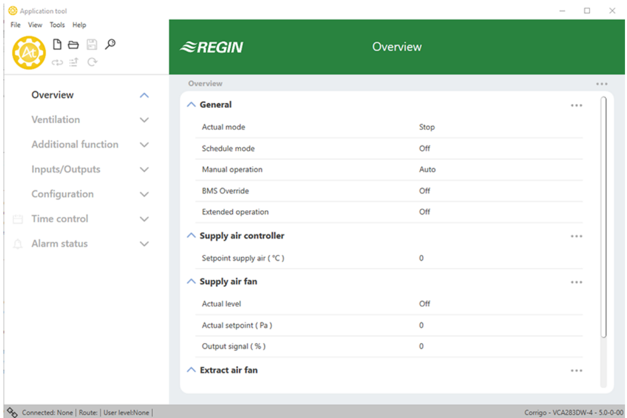
Bild 5-2 Application Tool Startbildschirm
