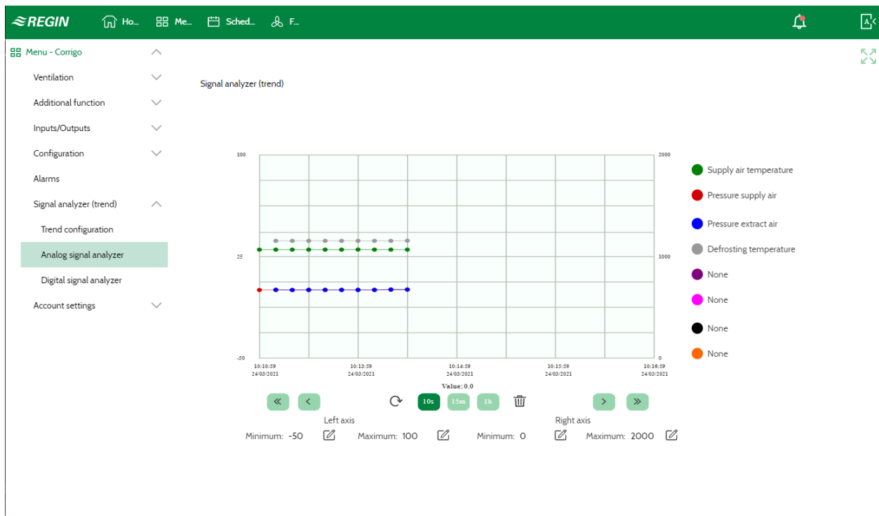
Bild 3-13 Signalanalysator, Analogsignal
