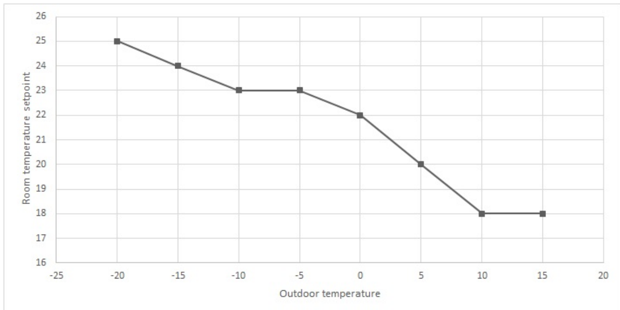
Bild 4-3 Temperatur-Kompensationskurve
