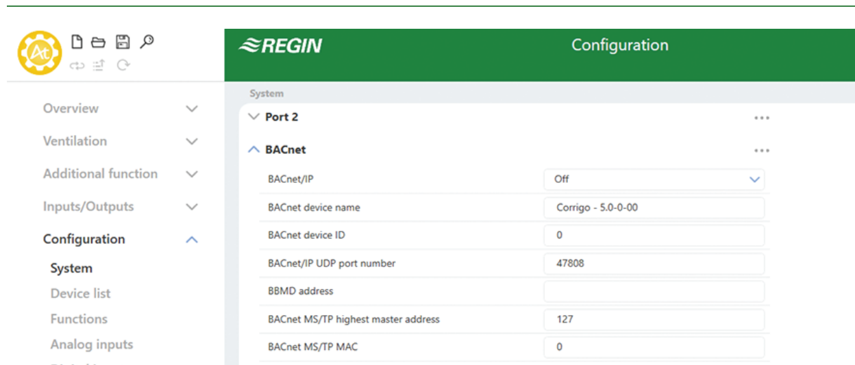
Bild 5-4 Alle BACnet Einstellungen
