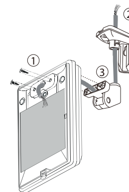
Fig. 3 Installation du détecteur sur le support
