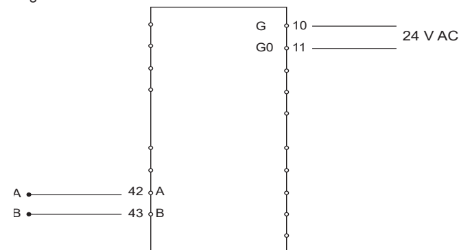
Bild 1 Verdrahtung
