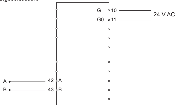
Bild 1 Verdrahtung
