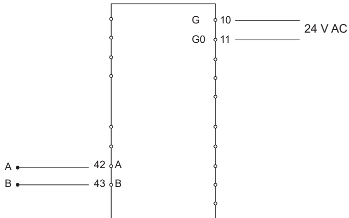
Bild 1 Verdrahtung
