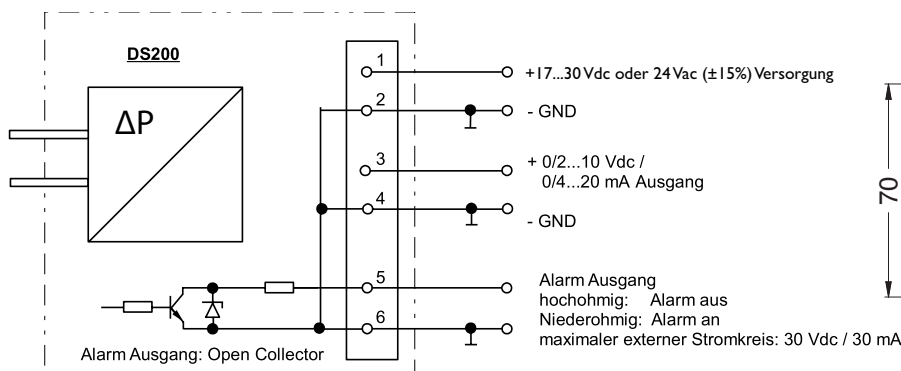
Anschlussschaltbild
