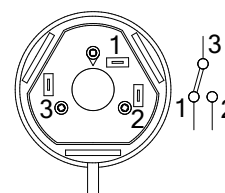
Anschlussschaltbild Druckschalter
